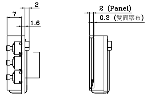
A-A'剖面圖
